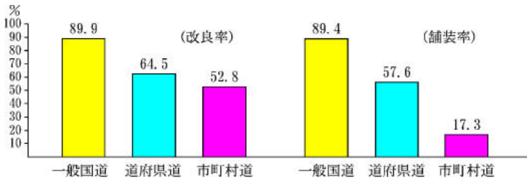
道路整備状況 (平成 14 年 4 月 1 日)
