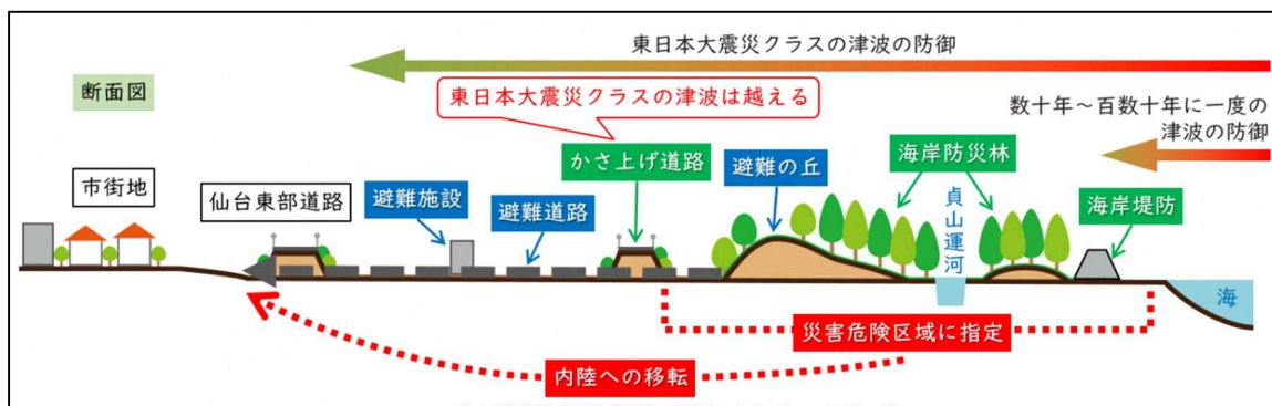
《津波多重防御断面図（イメージ）》
