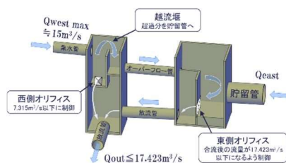
《二つのオリフィスによる流量制御の概要》
