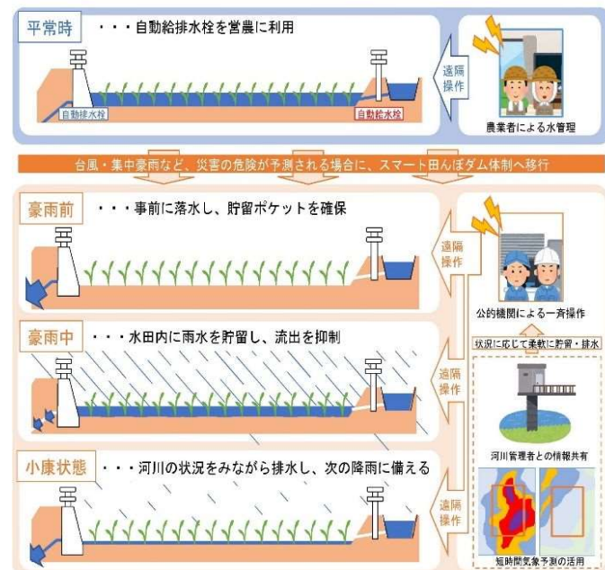
《スマート田んぼダムのイメージ》
