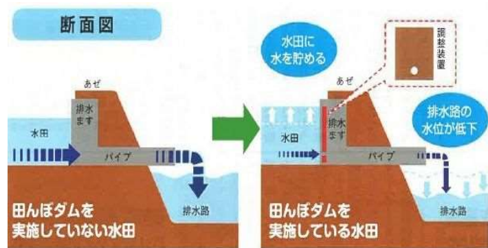
《田んぼダムのイメージ》
