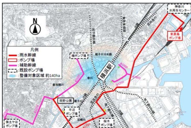
《エキサイトよこはま龍宮橋雨水幹線図》
